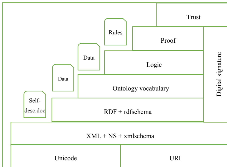
شکل ۱. ساختار وب معنایی (Berners-Lee, 2000)
